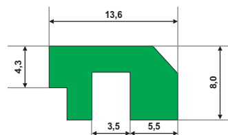
TYP: F1z | KOLOR: ZIELONY, BIAŁY | WAGA: 70 g/mb
