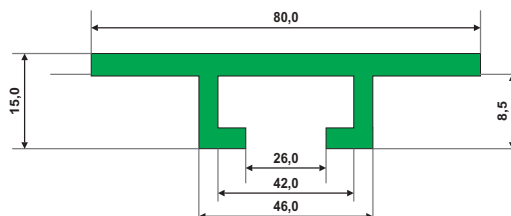
TYP: MTBz | KOLOR: ZIELONY, BIAŁY
