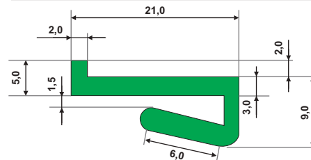
TYP: B6z | KOLOR: ZIELONY, BIAŁY | WAGA: 100 g/mb
