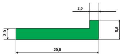
TYP: L1z | KOLOR: ZIELONY, BIAŁY | WAGA: 58 g/mb
