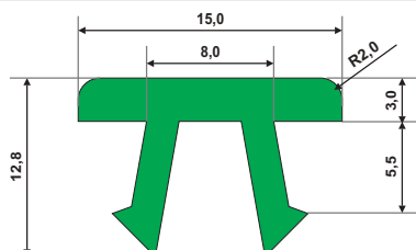
TYP: K2z | KOLOR: ZIELONY, BIAŁY | WAGA: 75 g/mb
